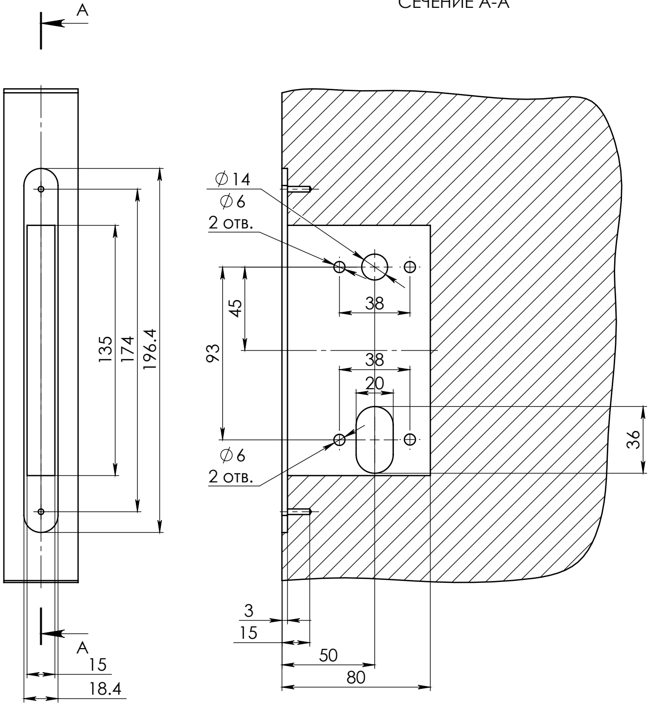
СЕЧЕНИЕ А-А
