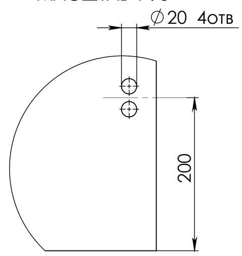
МЕСТНЫЙ В МАСШТАБ 1 : 5
