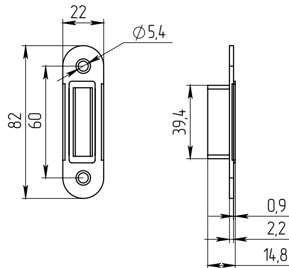
Ответная планка PRM-1
