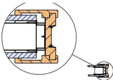
СЕЧЕНИЕ В-В
